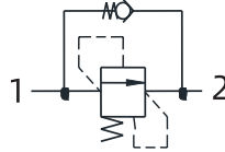
原理图 Symbol
